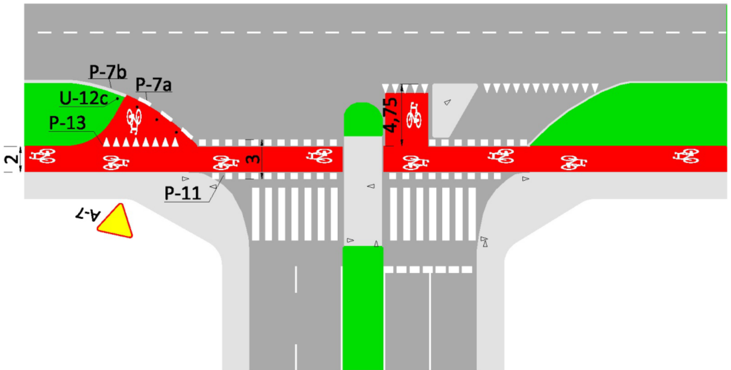
Rys. 20D. Droga dla rowerów i przejazdy dla rowerzystów ze śluzami do skrzyżowania (typu 3, pośrodku) i do skrzyżowania na drodze dla rowerów (typu 4, w lewym narożniku) umożliwiającymi bezpieczne pokonanie skrzyżowania na relacjach nie obsługiwanych drogami dla rowerów. Część oznakowania pionowego pominięto.
