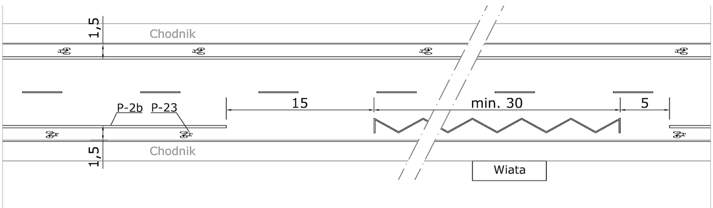
Rys. 6. Pas ruchu dla rowerów w rejonie przystanku zlokalizowanego na jezdni.
