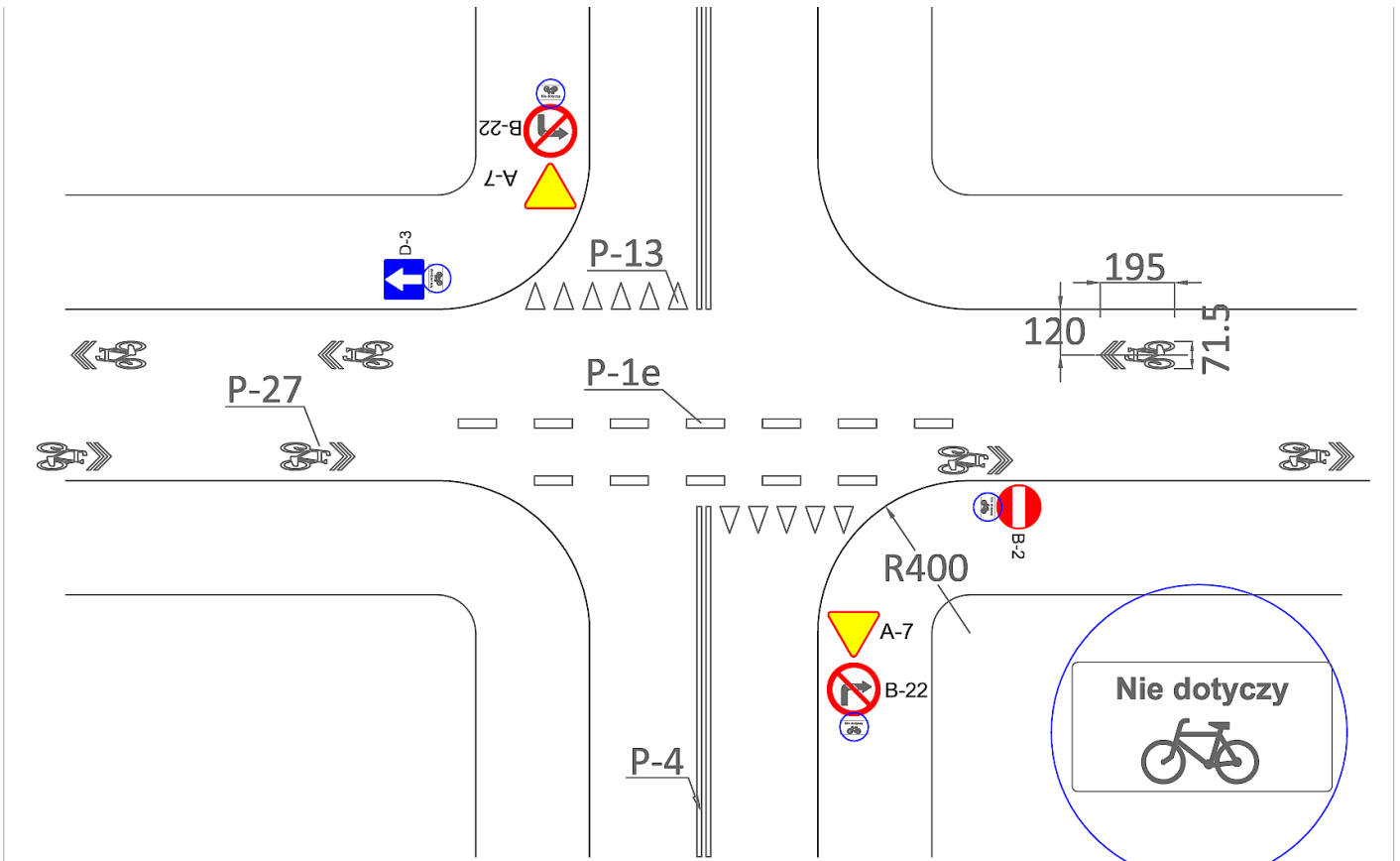
Rys. 4. Przykładowa organizacja dwukierunkowego ruchu rowerowego na jezdni jednokierunkowej – skrzyżowanie z ustalonym pierwszeństwem. Ruch „pod prąd” dopuszczony jest oznakowaniem poziomym P-27, znaki dla kierunku pod prąd umieszcza się zgodnie z opisem w tekście (punkt 4.3), wymiarowanie położenia dla kierunku zgodnego z ogólną organizacją ruchu przedstawiono na rysunku.
