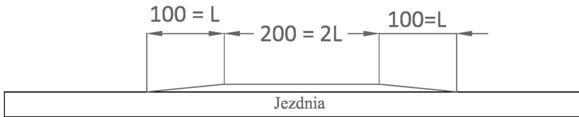
Rys. 1. Płyty pręga zwalniający – przekrój podłużny
