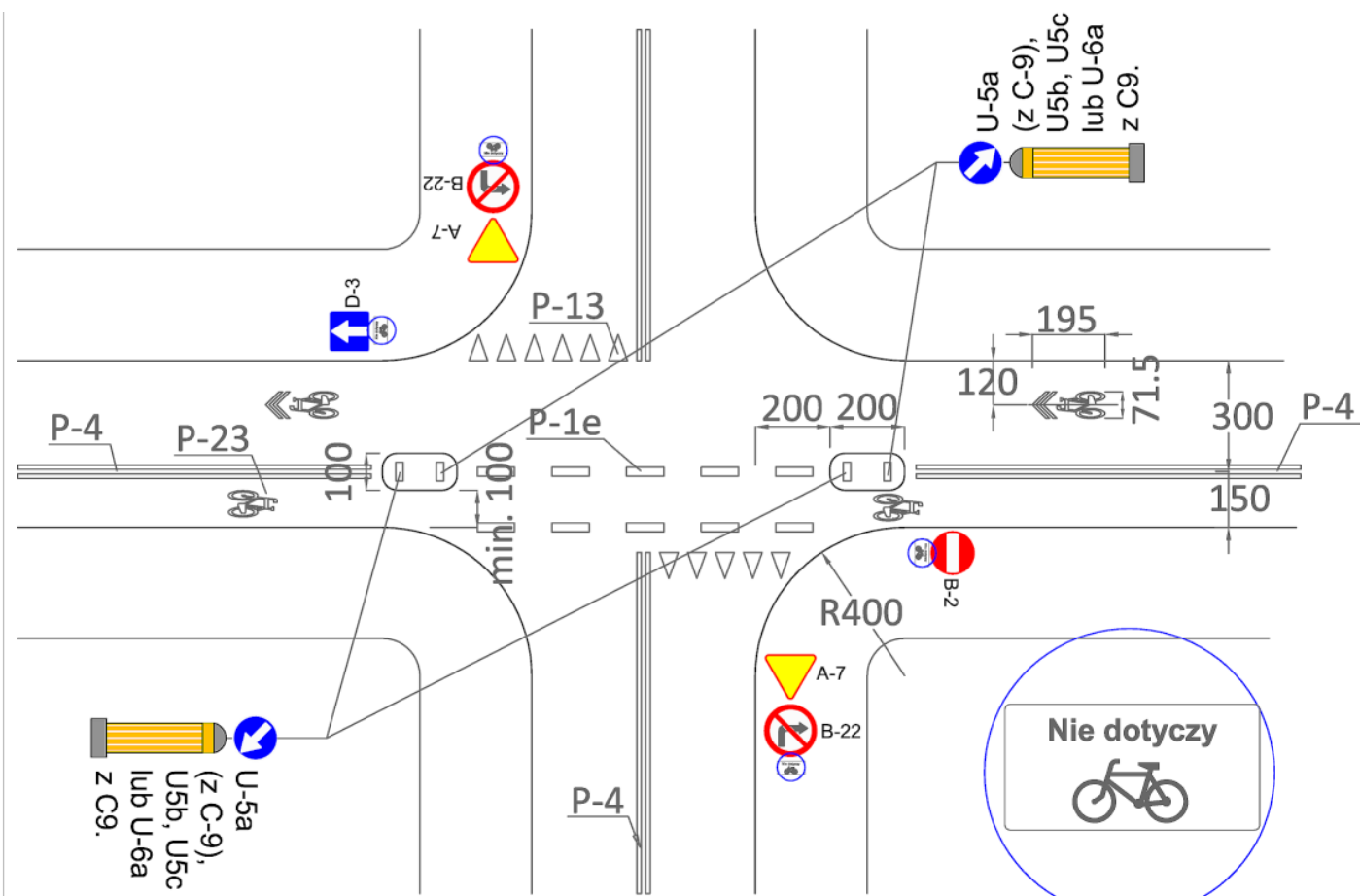
Rys. 10B. Przykład kontrapasa z wyspami dzielącymi na wlocach (porównaj z rys. 11).
