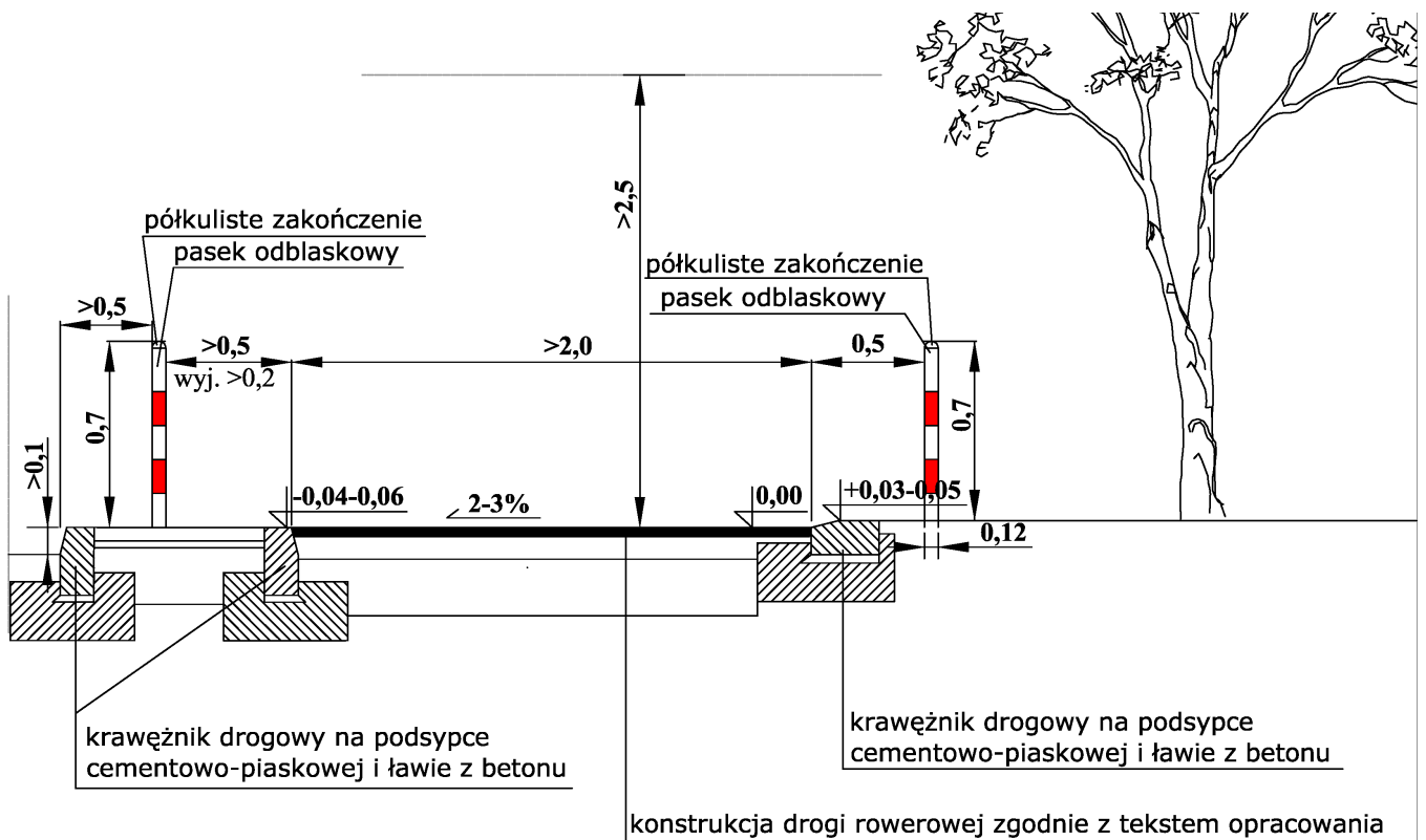
Rys. 12B. Inny przykład rozwiązania konstrukcyjnego drogi dla rowerów - przekrój poprzeczny dwukierunkowej drogi dla rowerów o nawierzchni bitumicznej, wariant zamknięty z obu stron krawężnikami drogowymi, w tym leżącym krawężnikiem drogowym oddzielającym ją od przylegającego chodnika (nieujęty na rysunku). Zastosowanie słupków U-12c jest opcjonalne.
