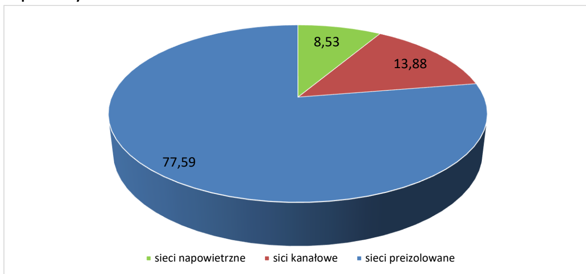
Wykres 10 Udział poszczególnych rodzajów sieci ciepłych w leszczyńskim systemie ciepłowniczym
