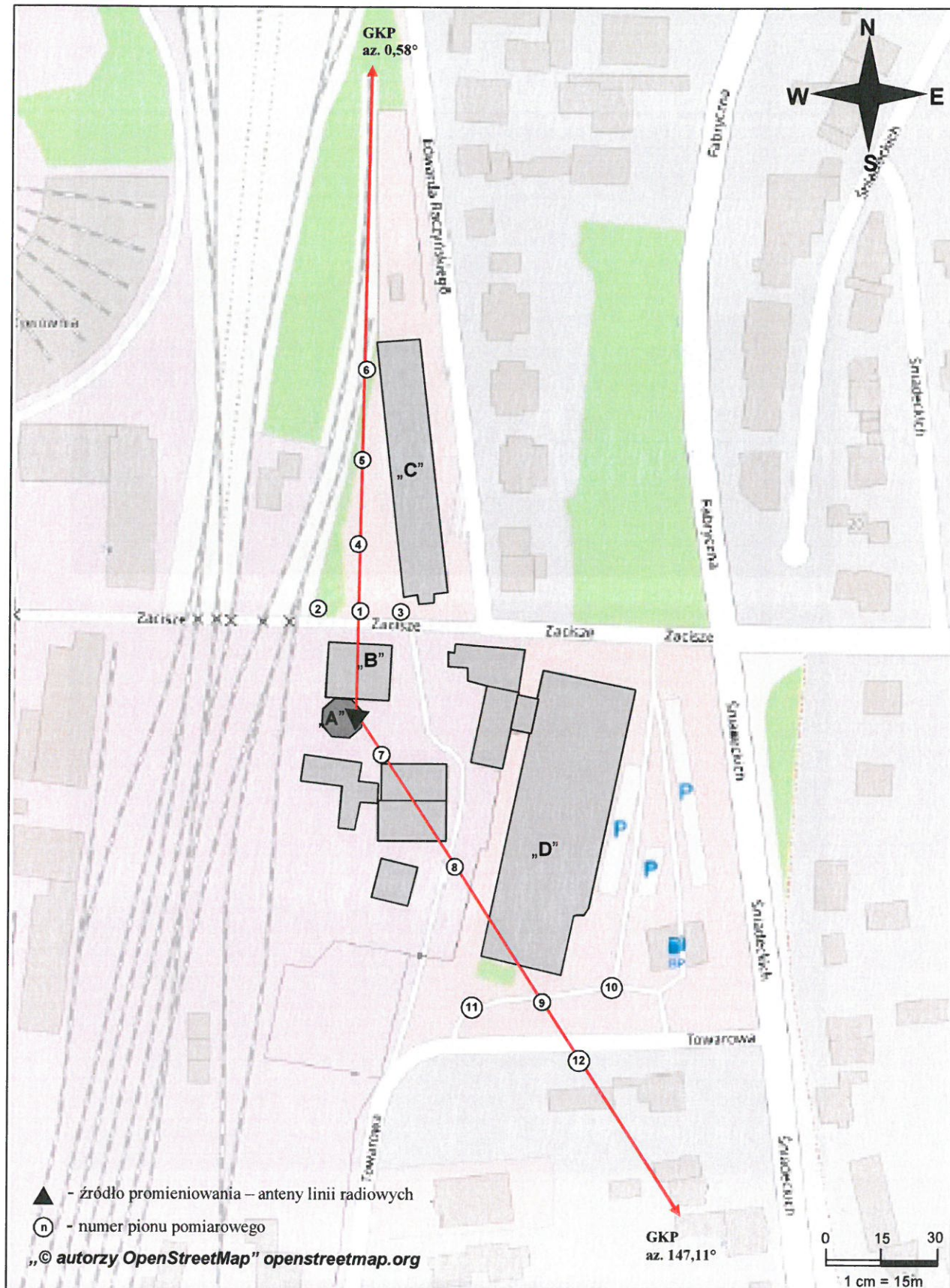
Rys. 1. Usytuowanie punktów i pionów pomiarowych w otoczeniu instalacji radiokomunikacyjnej Stacja Netia LESZB060-LESZM00157 Leszno, ul. Zaczysze 1B [działka nr 1/7 obręb Leszno].
