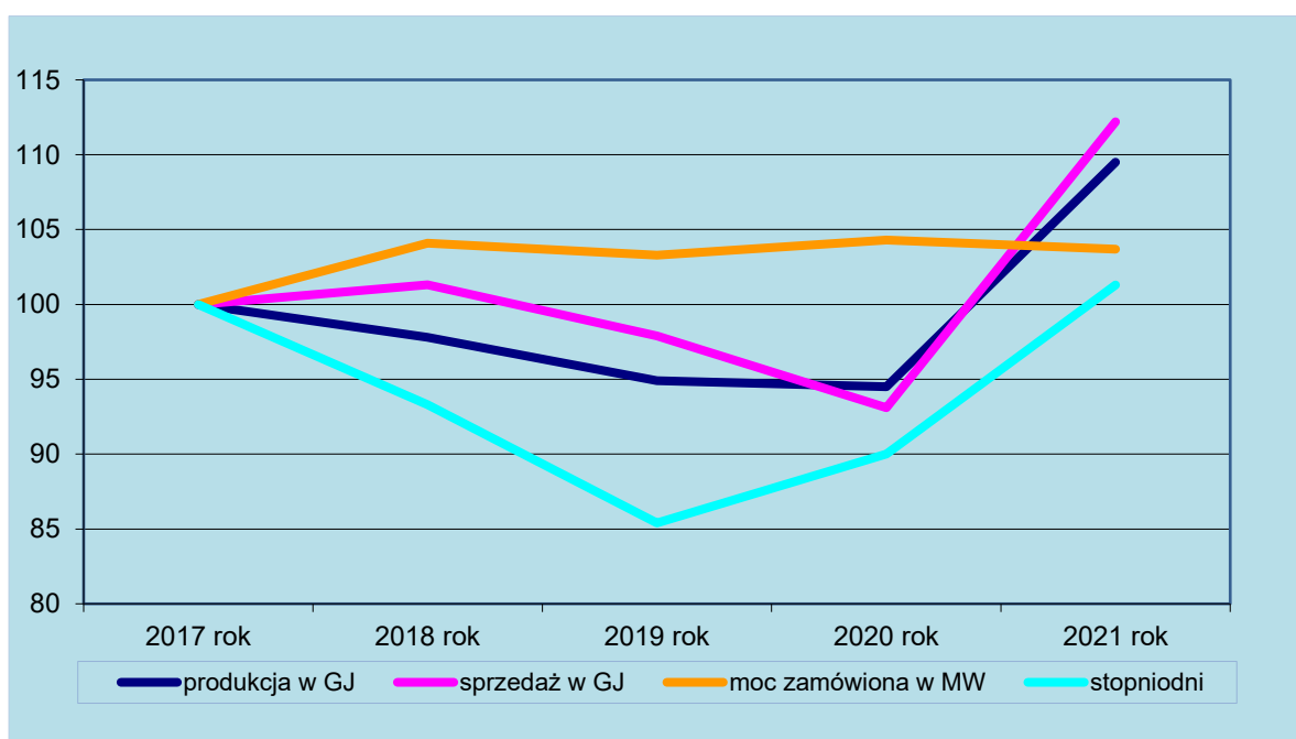
Wykres 11 Dynamika produkcji i sprzedaży energii cieplnej, mocy zamówionej i stopniodni w latach 2015-2021
