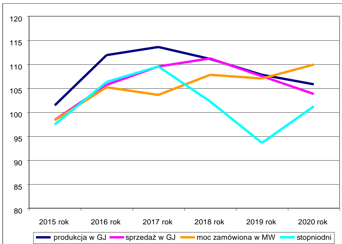
Wykres 11 Dynamika produkcji i sprzedaży energii cieplnej, mocy zamówionej i stopniodni w latach 2015-2020
