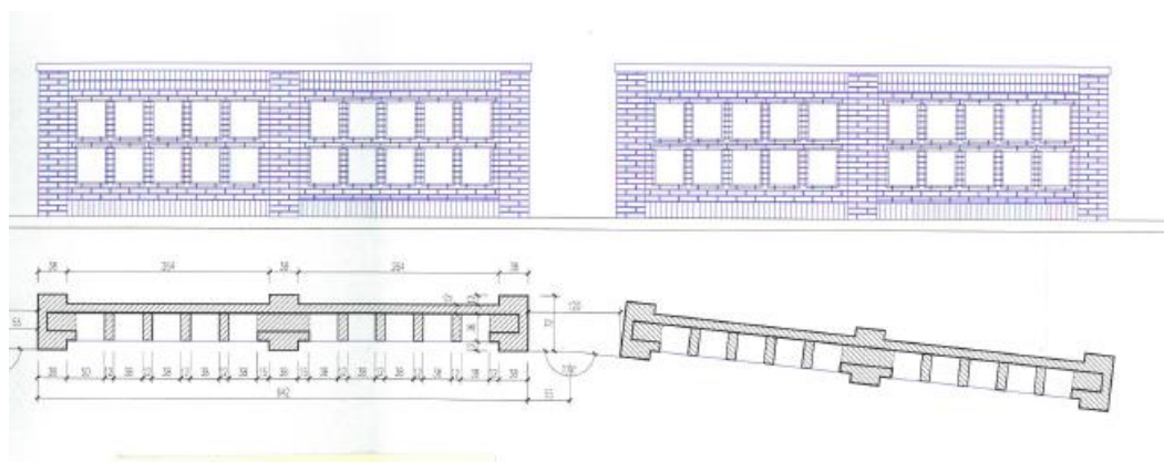
Rysunek 4 Projektowana ściana z niszami
